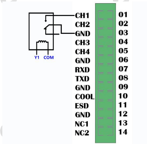
PLC 输出接线图:
