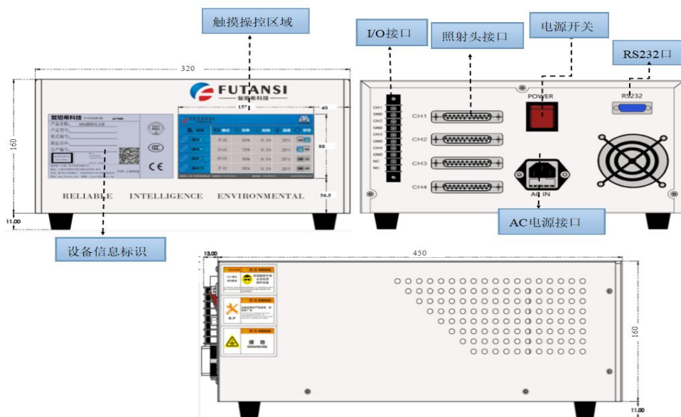
控制器外形尺寸图：
