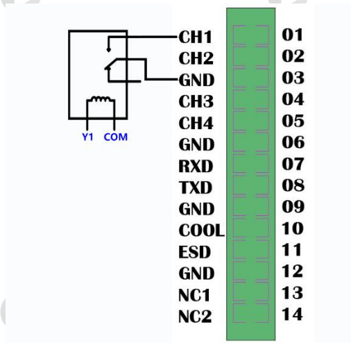
PLC 输出接线图:
